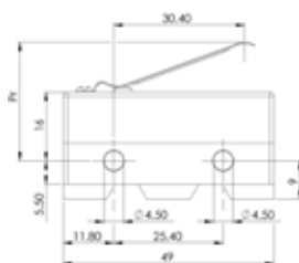
Type 2A : Simple Lever - Direct Action -
